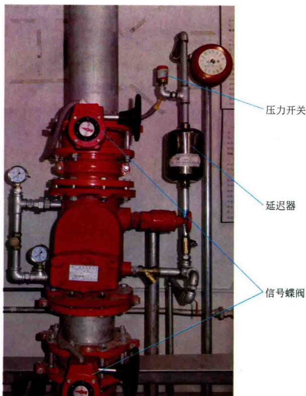
图5-9 湿式自动喷水灭火系统
