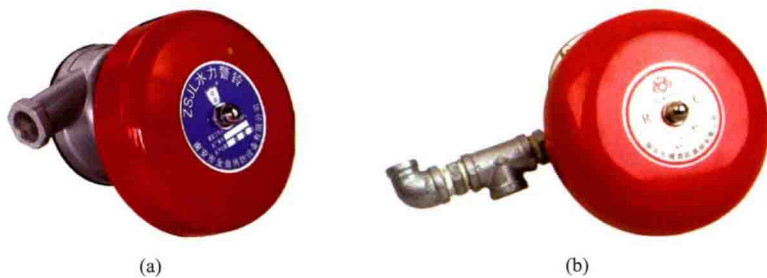
图 5-21 水力警铃
